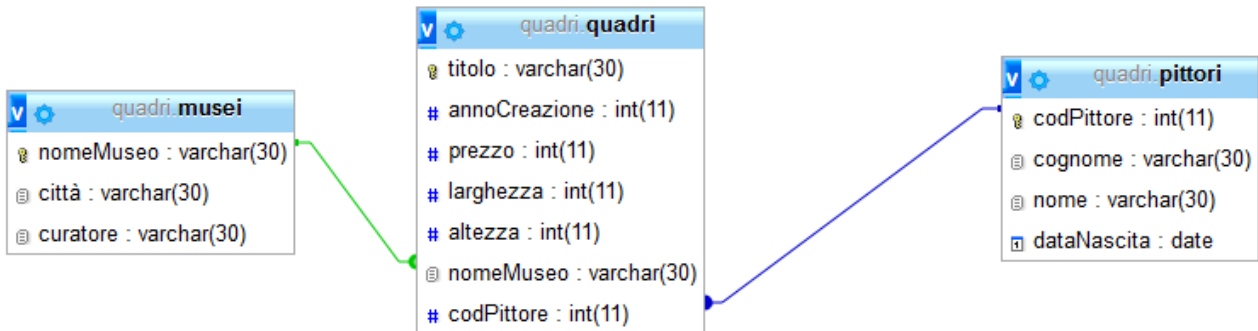
Figura 1 - mySQL
